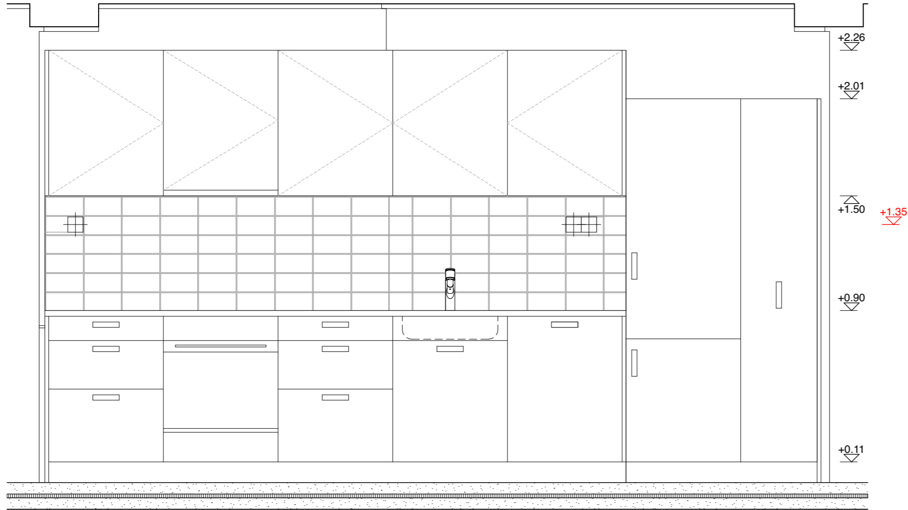
Ansicht B-B
