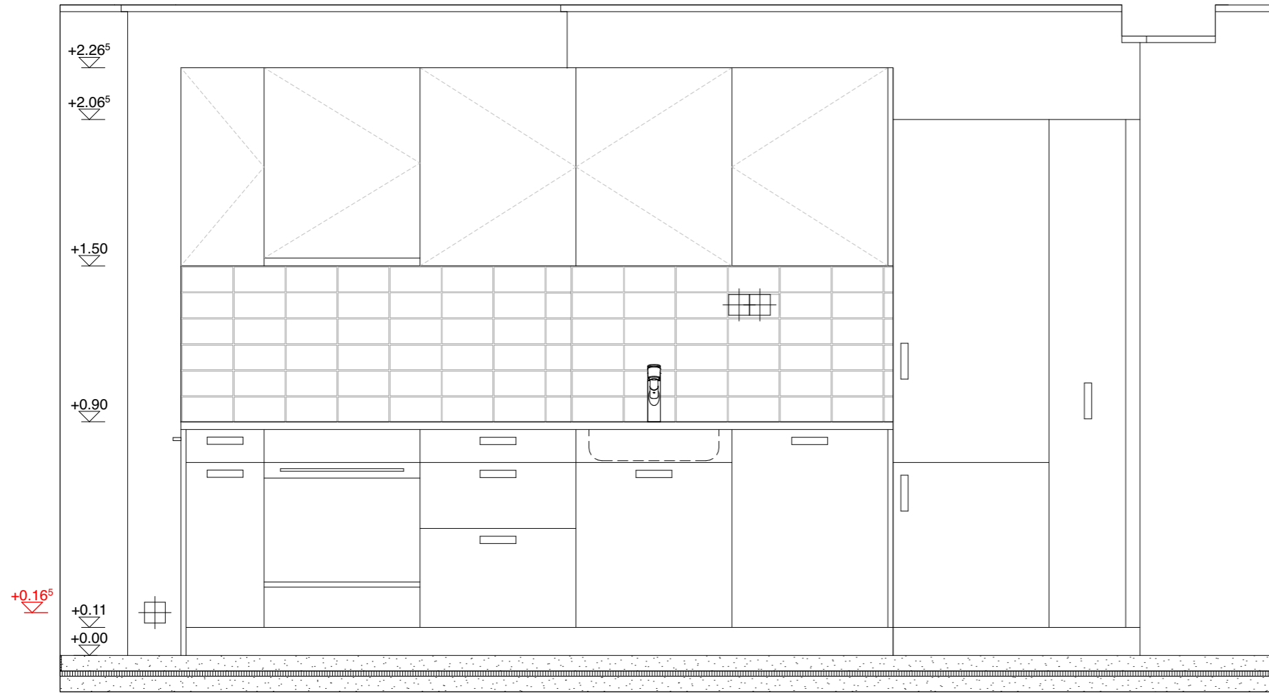
Ansicht
