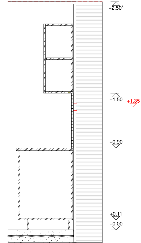
Schnitt B-B
