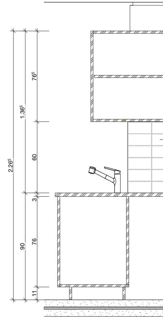
Schnitt A-A
